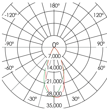
— C0 - C180 — C90 - C270 Unidad: cd
