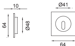
SD221 rosetta incasso foro chiave sliding door handle key hole
