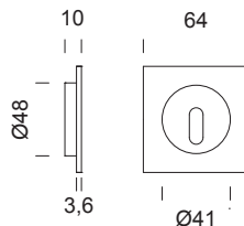
SD223 set maniglie incasso foro chiave con frontale sliding door handle set key hole with flush pull hole
