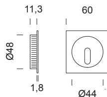
SD522 set maniglie incasso foro chiave con frontale sliding door handle set key hole with flush pull hole
