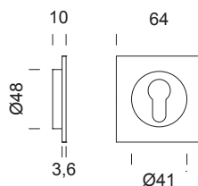
SD222Y set maniglie incasso foro yale con frontale sliding door handle set yale hole with flush pull hole
