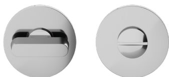
FINE RDN20+A set nottolino su rosetta turn & release set on rose 50x4mm - FINE
