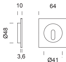
SD223 set maniglie incasso foro chiave con frontale sliding door handle set key hole with flush pull hole
