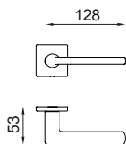
LP14 senza bocchetta without escutcheon
