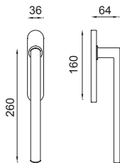
LC50 maniglione su placca cieca con placchetta incasso pull handle on blind plate with sliding door handle
