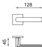
LC14 senza bocchetta without escutcheon
