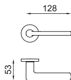
LP12 senza bocchetta without escutcheon
