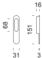
LP51 maniglione accoppiato su placca Yale pull handle set on Euro profile plate
