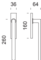
LC60 maniglione su placca cieca con placchetta incasso pull handle on blind plate with sliding door handle
