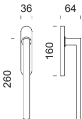
LC50 maniglione su placca cieca con placchetta incasso pull handle on blind plate with sliding door handle
