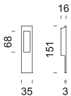
LC61 maniglione accoppiato su placca Yale pull handle set on Euro profile plate
