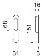
LC51 maniglione accoppiato su placca Yale pull handle set on Euro profile plate
