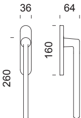
LP50 maniglione su placca cieca con placchetta incasso pull handle on blind plate with sliding door handle
