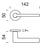
LP12 senza bocchetta without escutcheon
