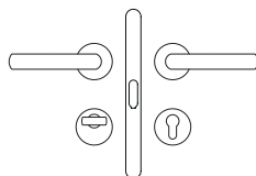
sistema Vertical con pomolo per cilindro Vertical system with knob for cylinder
